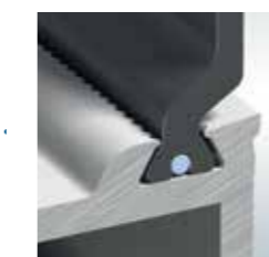
Cavità con profilo termoisolante insulbar inserito
