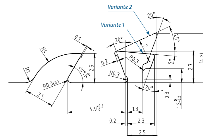
Cavità di alluminio estrusa
