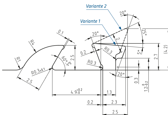
Cavità di alluminio estrusa
