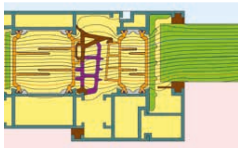
U_f -Wert = 1,18 W/m 2 K: identisches Fenstersystem mit insulbar LI
